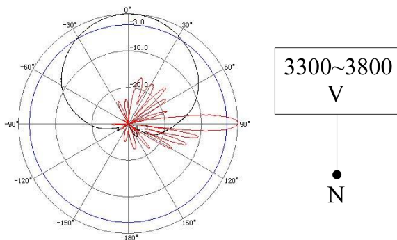
典型方向图:
